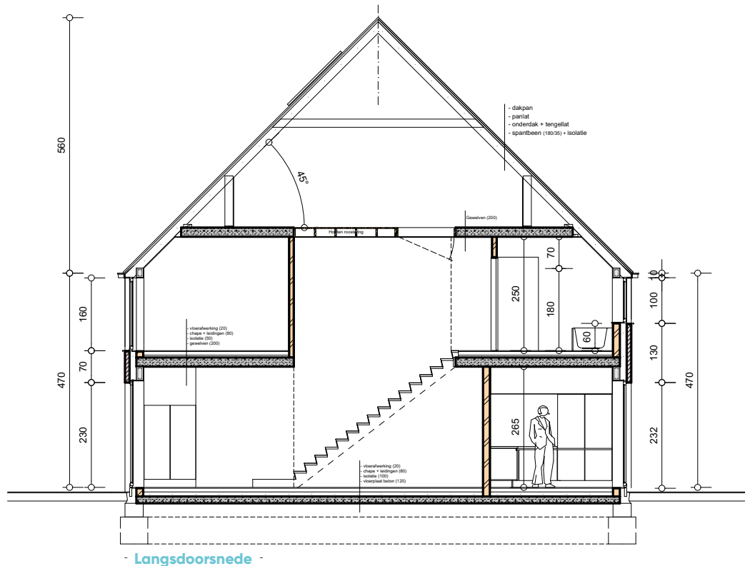
- Langsdoorsnede -
